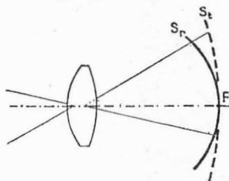
FIG. 26. ASTIGMATIC FOCAL PLANES
