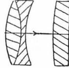
FIG. 76. ALDIS ANASTIGMAT, F/6
