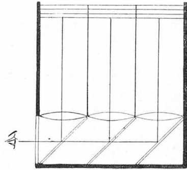
FIG. 217. CHROMSCOPE (Ducos Du Hauron)
