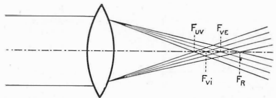
FIG. 18. CHROMATIC ABERRATION
