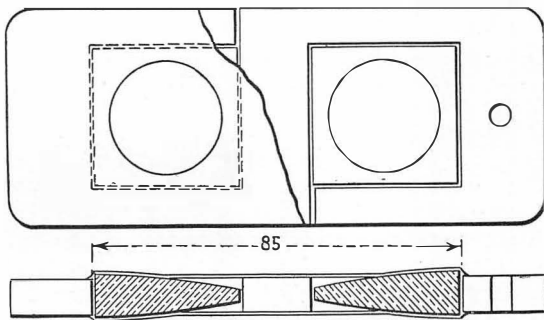
FIG. 208. STEREOSCOPIC BINOCLE (Buguet)
